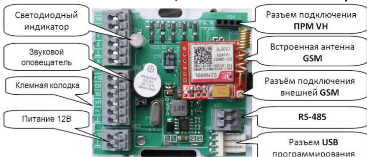
Размещение элементов на плате прибора
